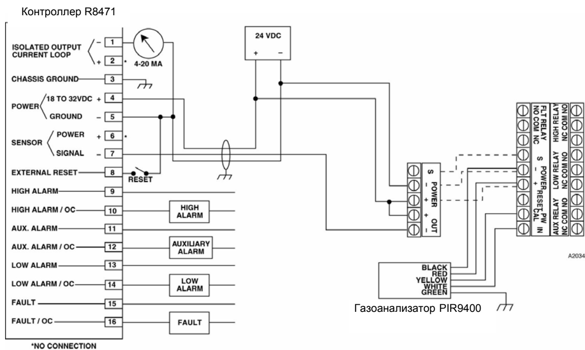
Рис. 13. Типовая схема подключения контроллера U9500 с газоанализатором PIR9400 и контроллером R8471, с неизолированным токовым выходом.
