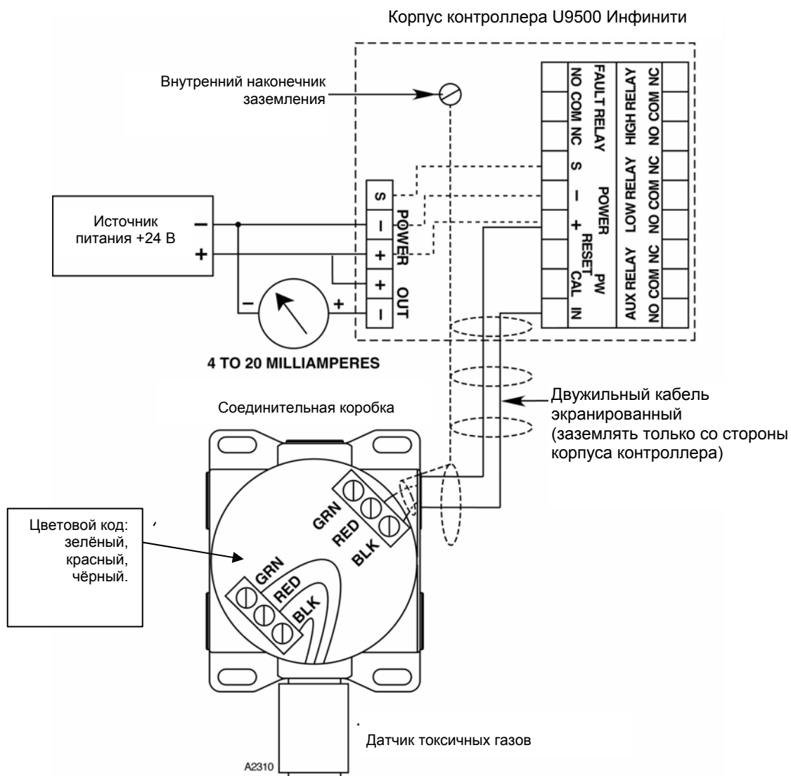
Рис. 17. Выносная установка датчиков токсичных газов* и кислорода с контроллером U9500.
