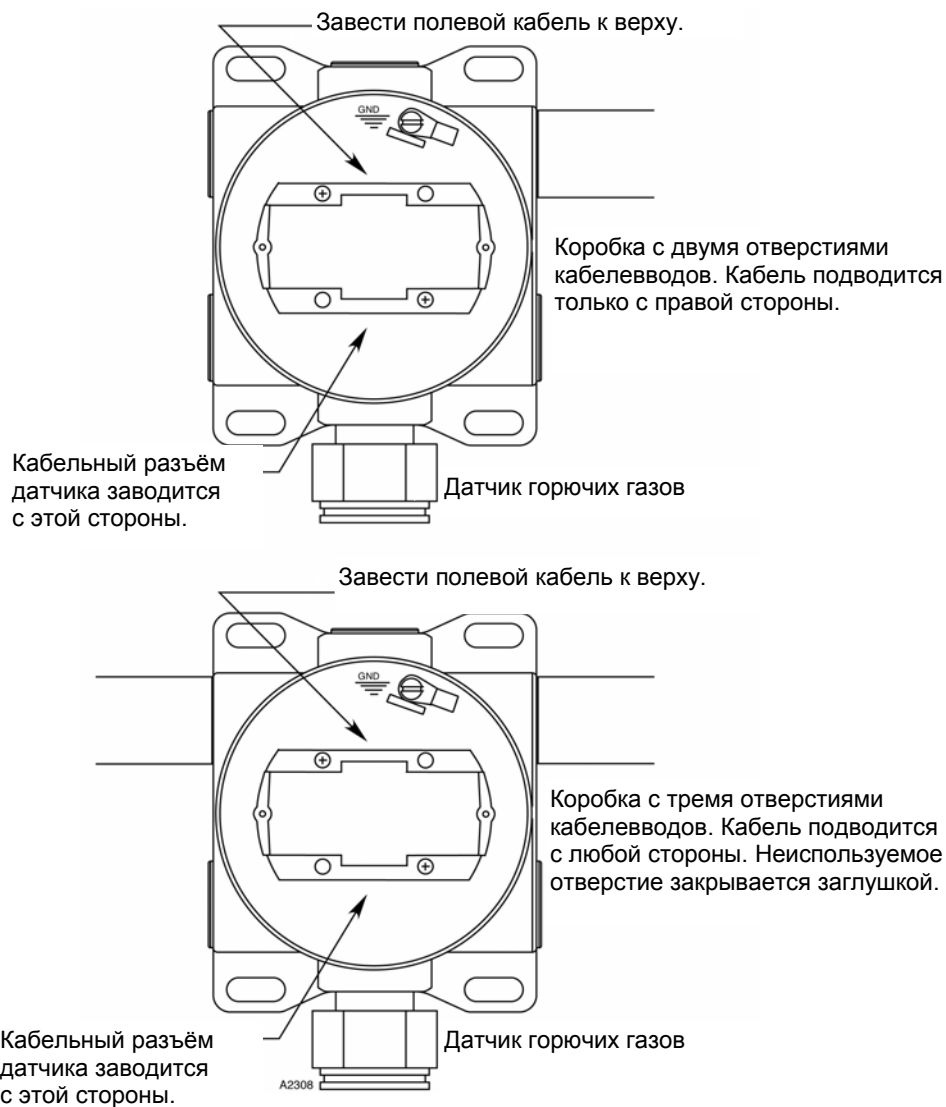
Рис. 4. Кабельные входы концевой разводки.
