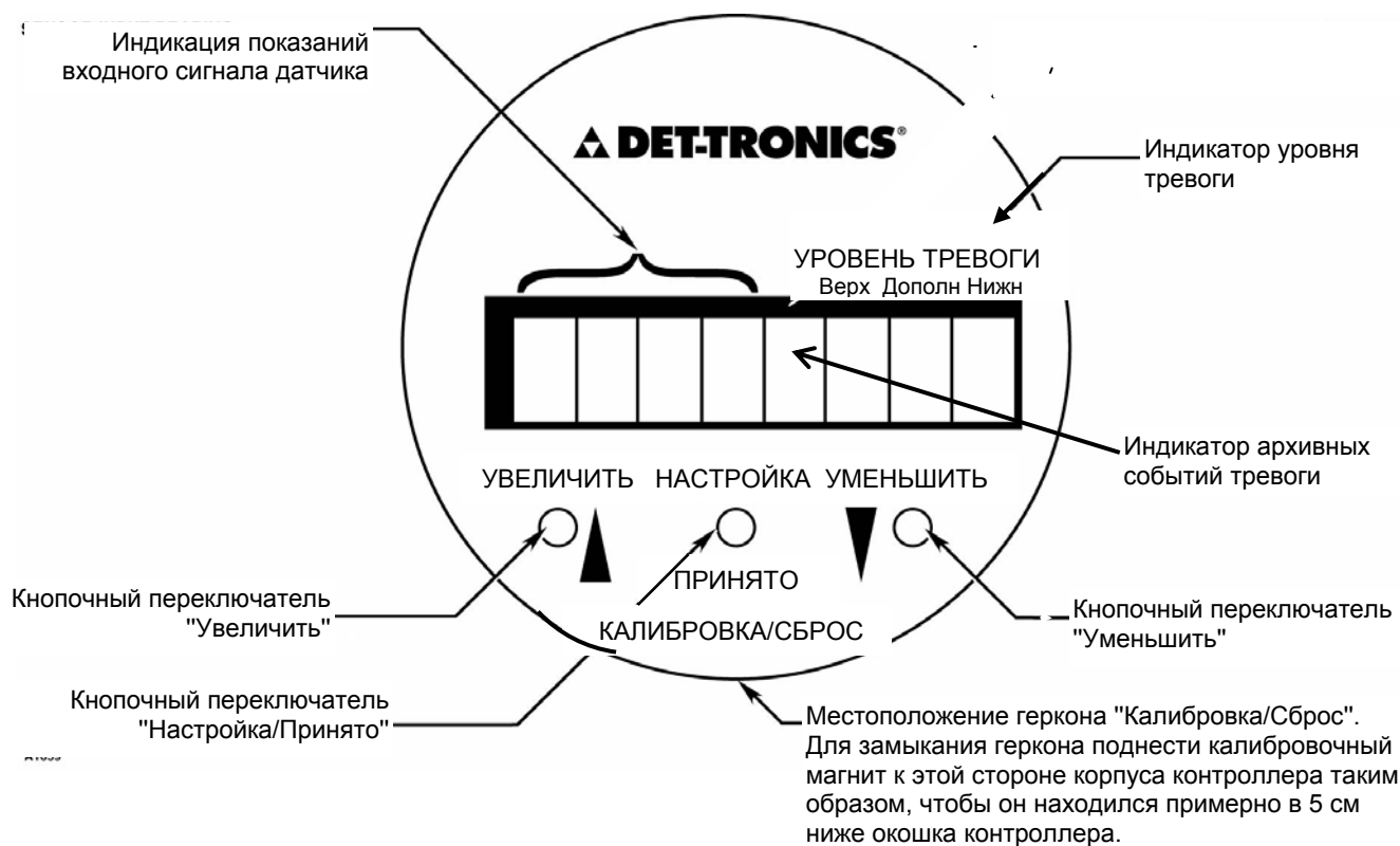
Рис. 19. Индикаторы и органы управления контроллера.
