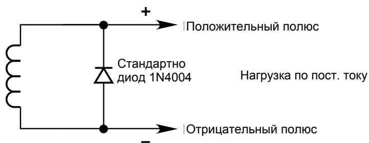
Рис. 11. Подавление переходных процессов на индуктивных нагрузках.
