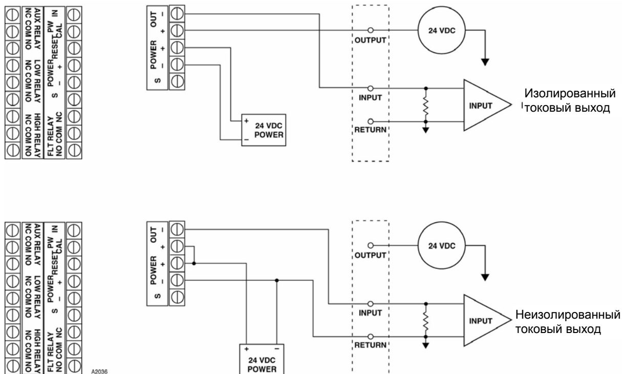
Рис. 14. Типовая схема подключения контроллера U9500 с ПЛК, с изолированным и неизолированным токовыми выходами.
