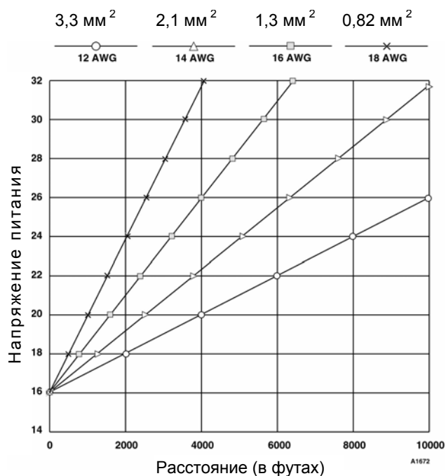
Рис. 3. Требования к сечению проводов питания для контроллеров с релейными выходами при работе с горючими газами и датчиком MOS H 2 S.
