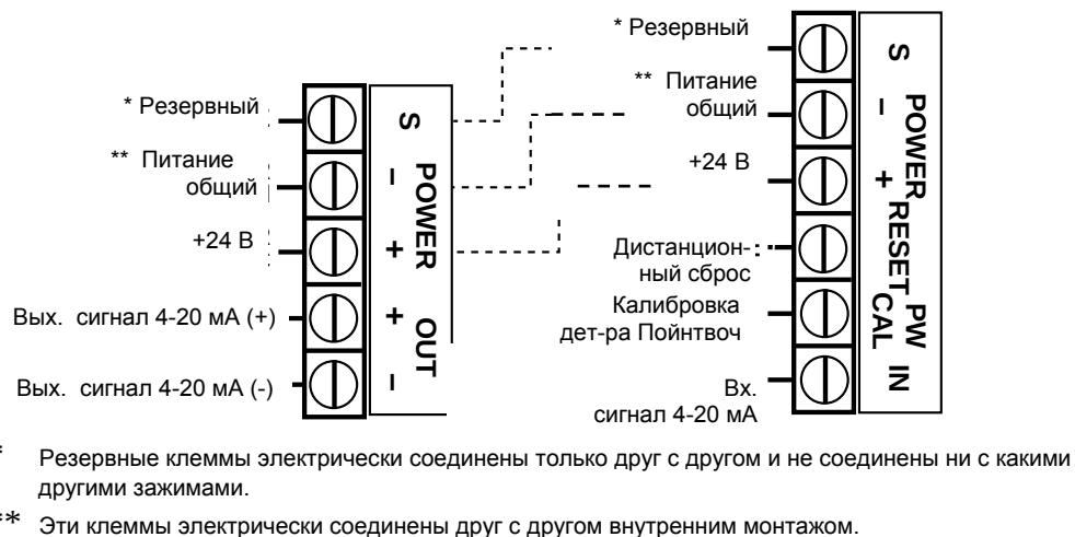
Рис. 6. Блок контактных зажимов контроллера без реле.
