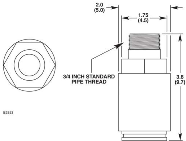
Рис. 5. Габаритные размеры газоанализатора NTMOS в дюймах (см).
