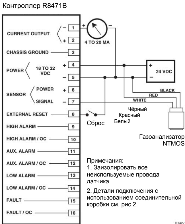
Рис.4. Газоанализатор NTMOS, подключённый непосредственно к контроллеру R8471B.
