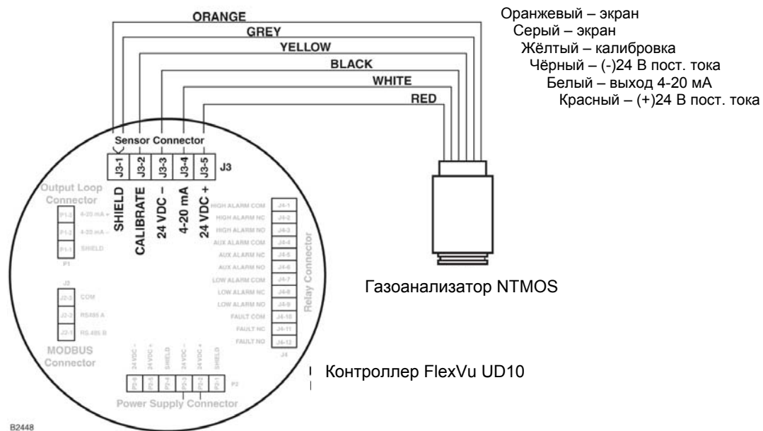
Рис.1. Газоанализатор NTMOS, подключённый непосредственно к контроллеру FlexVu UD10.
