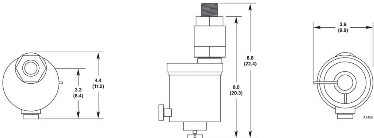
Рис. 6. Габаритные размеры газоанализатора NTMOS с ампульным калибровочным набором и установленной смесительной камерой в дюймах (см).
