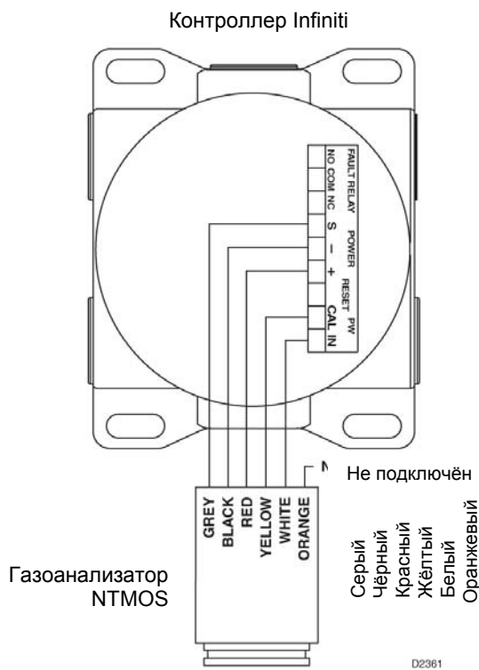
Рис.3. Газоанализатор NTMOS, подключённый непосредственно к контроллеру U9500 Infiniti.
