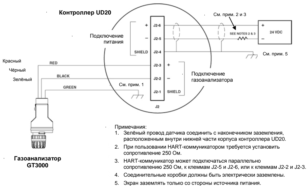
Рис. 8. Газоанализатор GT3000, подключенный непосредственно к контроллеру UD20.
